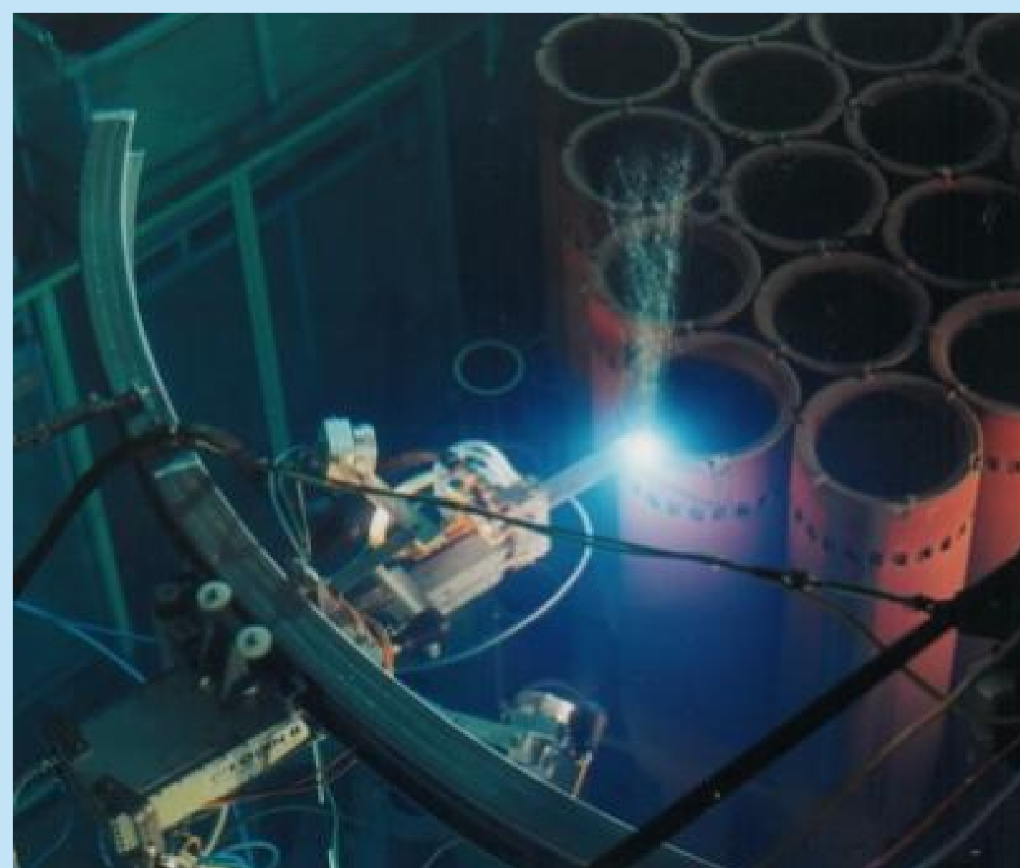
Unterwasser-Lichtbogenschneiden
