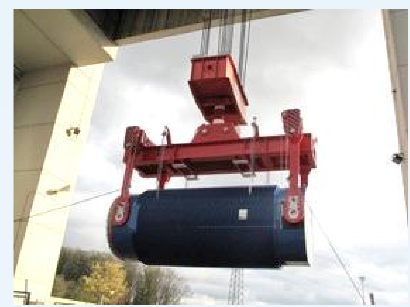
Ausschleusen aus dem Reaktorgebäude
