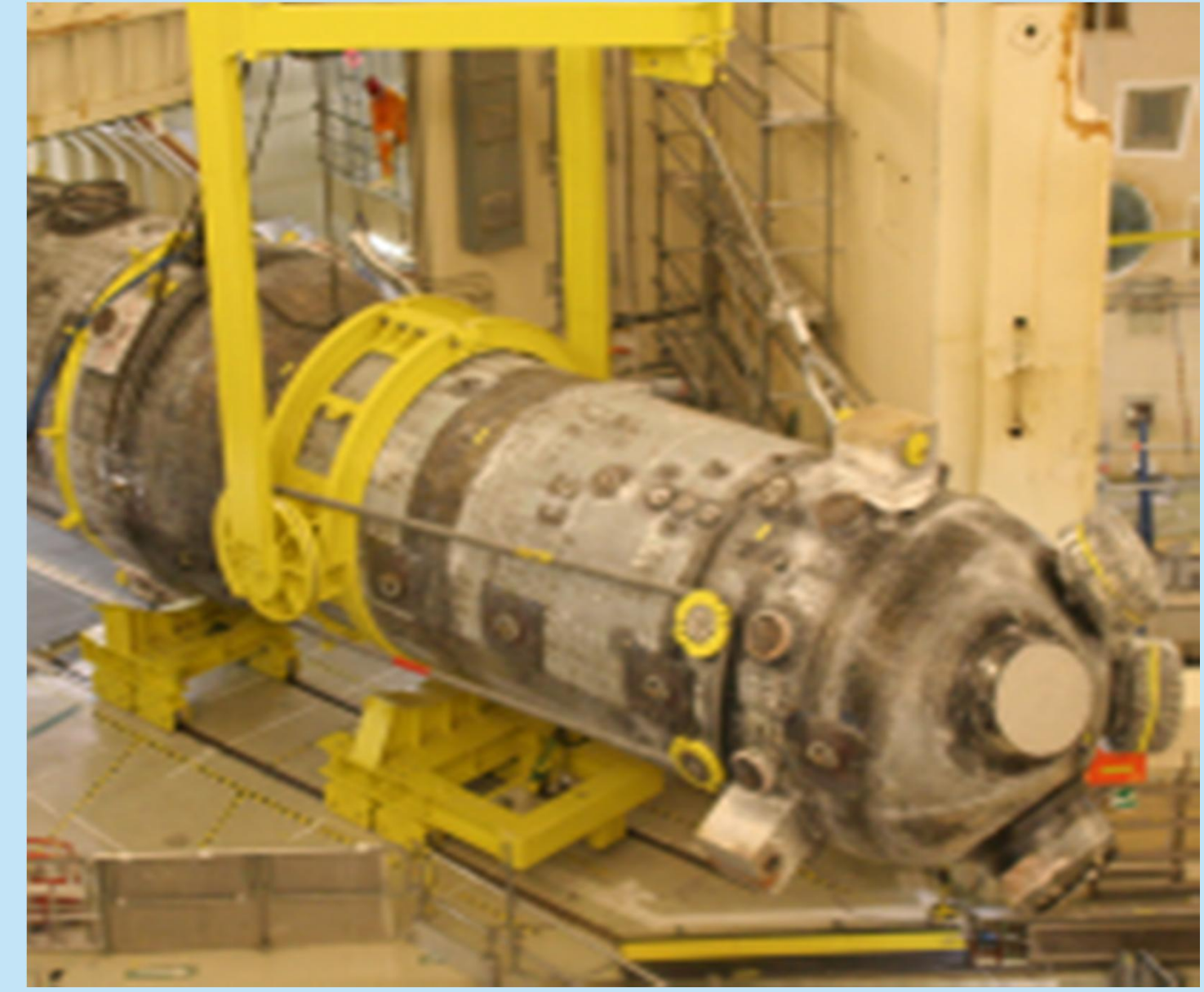
Ausbau und externe Bearbeitung
