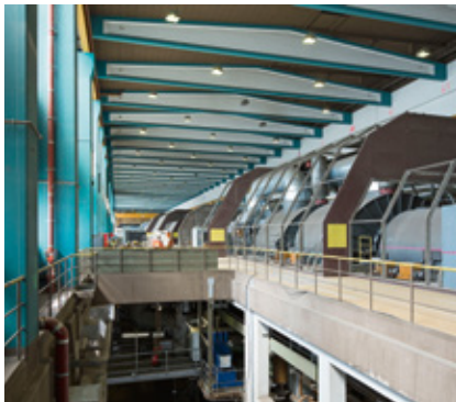
Blick in die Maschinenhalle mit 600-Megawatt-Turbosätzen
