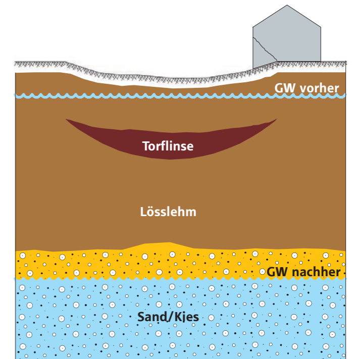
Bodenaufbau im Bereich des obersten freien Grundwasserspiegels GW = oberster Grundwasserspiegel
